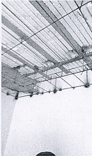
شکل ۳- ساپورت گیری نامناسب از تیرچه و تخریب آنها
